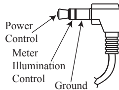
Figure 09– Power control (trigger) mini plug
